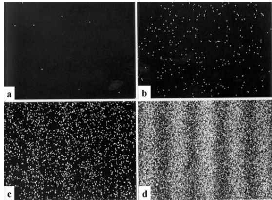
partikkelbølger
