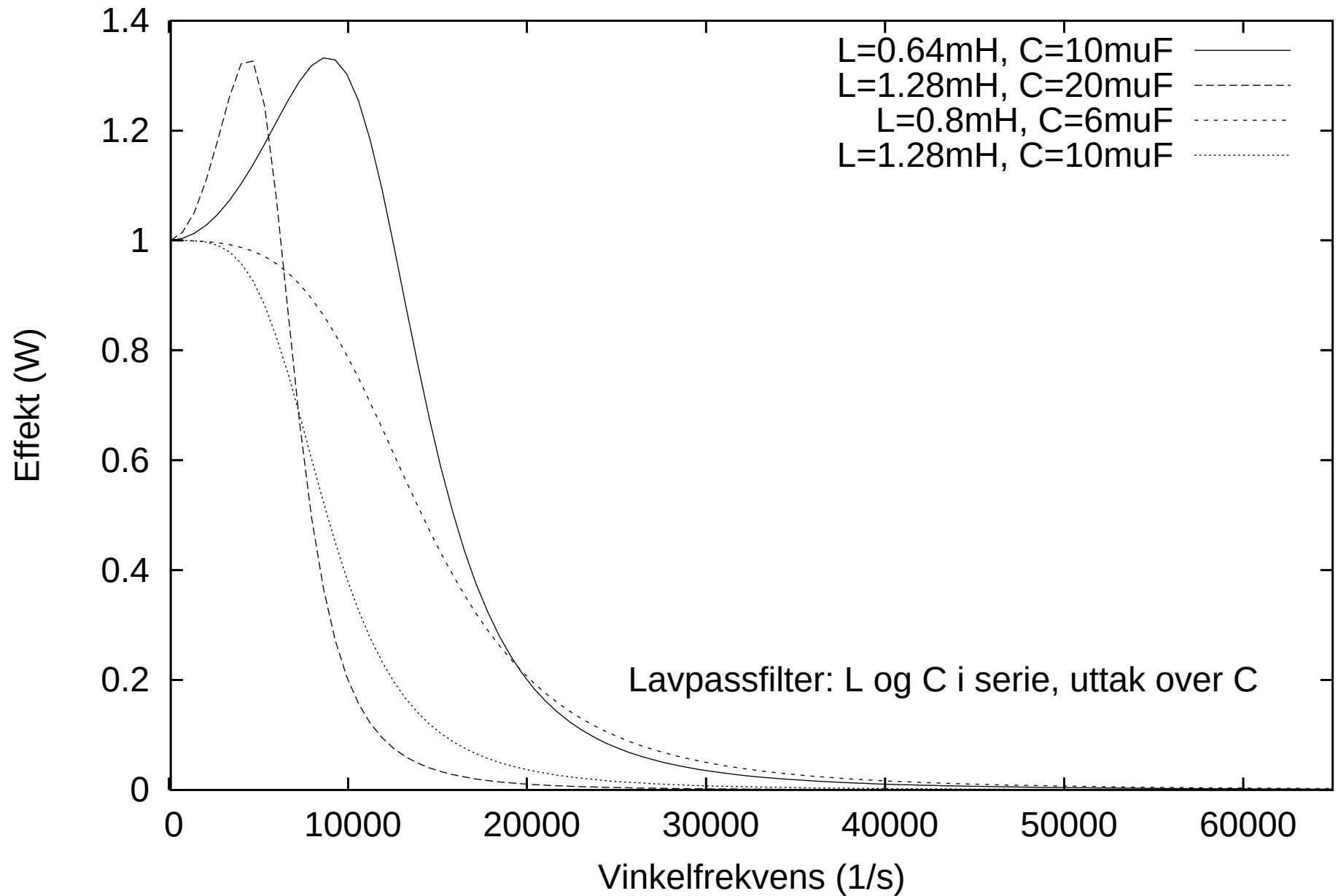
Effekt til bass med R=8\ \Omega og V_{in}=4\ \text{V}
