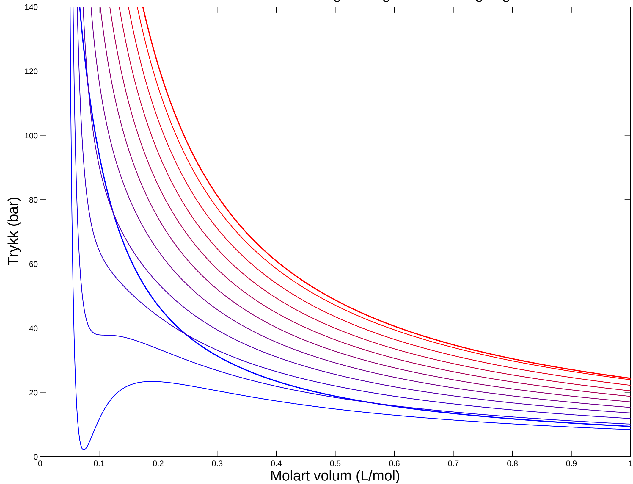
Isotermmer: van der Waals og ideell gass tilstandsligning
