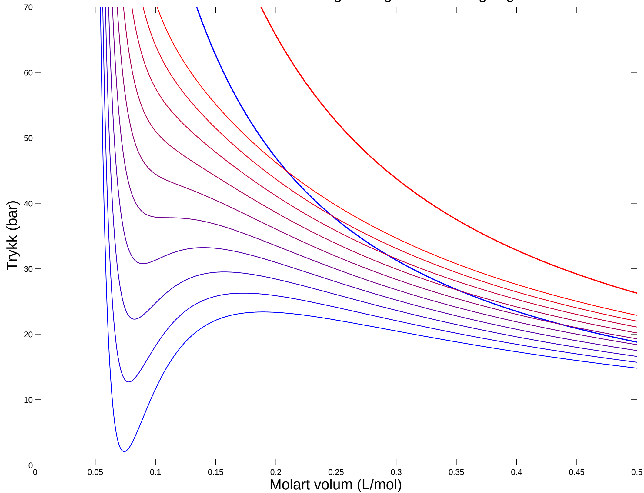
Isotermes: van der Waals og ideell gass tilstandsligning
