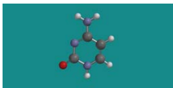
Cytosine
